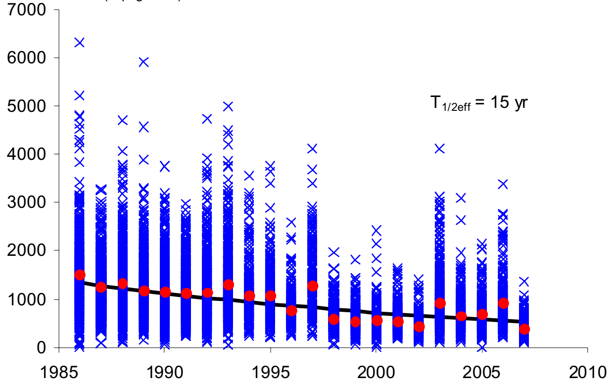
^{137}\text{Cs} in moose ( \text{Bq kg}^{-1} f.w.)
